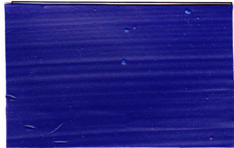
BLEU
